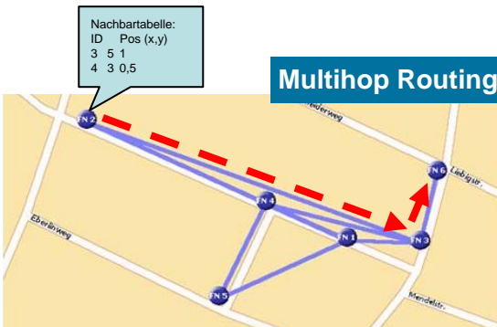
Greedy Packet Routing: Sender wählt den Knoten, der der Position des Ziels am nächsten ist. Kein Aufbau und Verwalten von Routen; Effiziente Datenübertragung auch bei hochmobilen Knoten.
